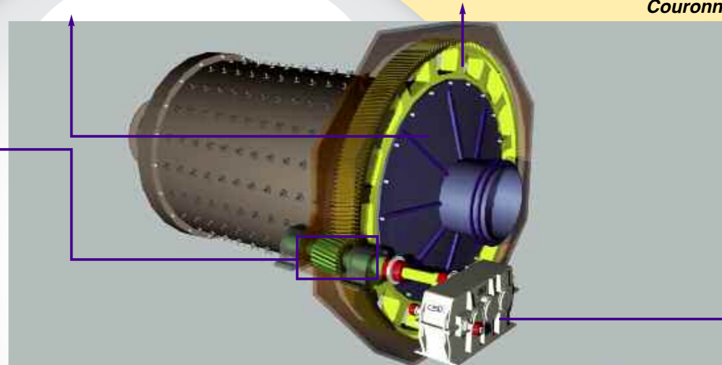
ATTAQUE LATÉRALE
